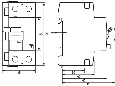
Dibujo acotado Vista de grupos
