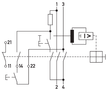
Esquema de conexiones
