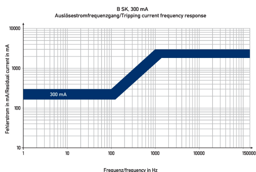
Diagramme Fehlerstromschutzschalter DFS 4 080-4/0,30-B SK R HD
