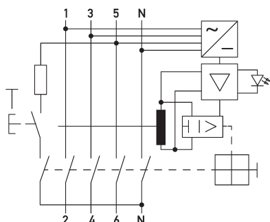
Schaltungsbeispiel Fehlerstromschutzschalter DFS 4 080-4/0,30-B SK R HD
