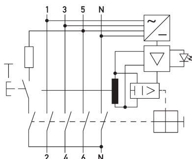
Schaltungsbeispiel Fehlerstromschutzschalter DFS4 080-4/0,30-B NK R HD
