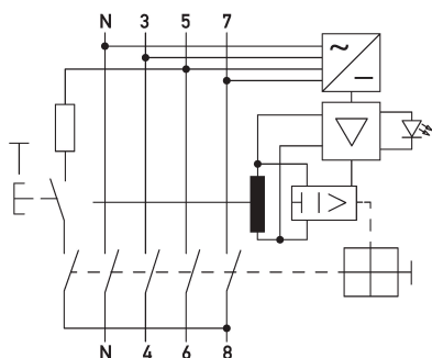
Schaltungsbeispiel Fehlerstromschutzschalter DFS 4 080-4/0,30-B SK V500
