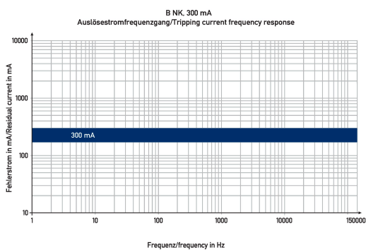
Curva característica B NK 300 mA
