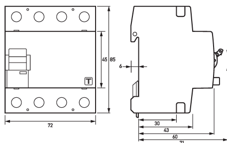
Dibujos acotados Interruptores diferenciales DFS 4 A V500, 4 polos
