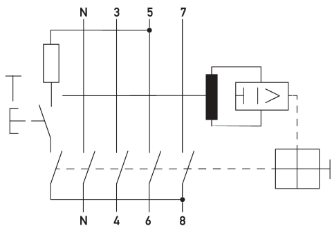
Ejemplo de cableado Interruptores diferenciales DFS 4 A V500, 4 polos
