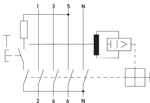
Ejemplo de cableado Interruptores diferenciales DFS 4 080-4/0,30-A R HD
