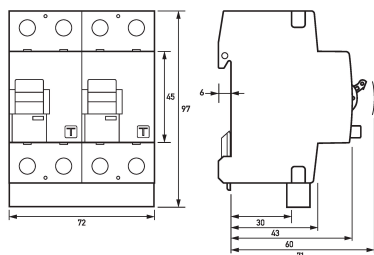
Maßzeichnung Gruppenansicht
