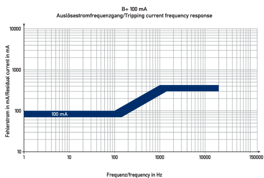
Diagramme Fehlerstromschutzschalter DFS 4 080-4/0,10-B+
