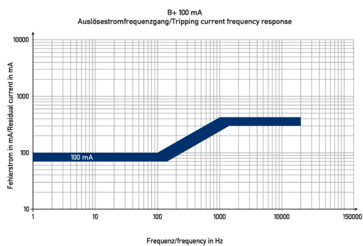
Diagramme Fehlerstromschutzschalter DFS 2 080-2/0,10-B+
