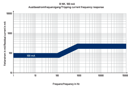
Curva característica B NK 100 mA
