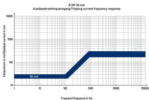
Diagramme Fehlerstromschutzschalter DFS 4 080-4/0,03-B NK HD
