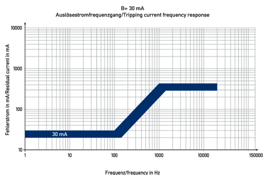
Diagramme Fehlerstromschutzschalter DFS 2 080-2/0,03-B+
