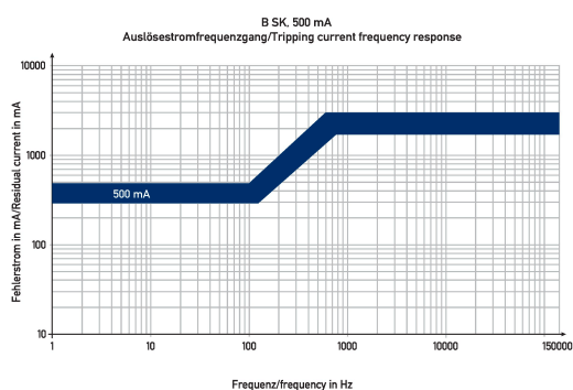
Diagramme Fehlerstromschutzschalter DFS 4 063-4/0,50-B SK S V500
