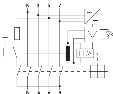
Schaltungsbeispiel Fehlerstromschutzschalter DFS 4 063-4/0,50-B SK S V500
