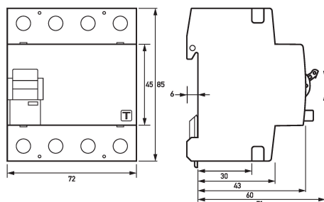
Maßzeichnung Fehlerstromschutzschalter DFS 4 063-4/0,50-B SK S V500
