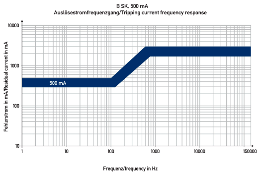
Diagramme Fehlerstromschutzschalter DFS 4 063-4/0,50-B SK MI R HD
