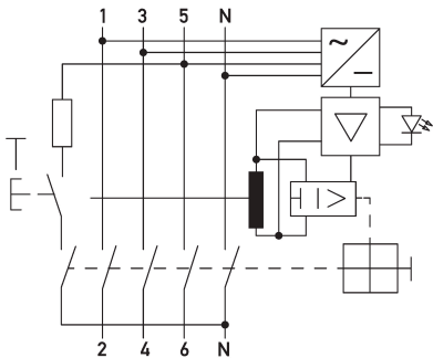
Schaltungsbeispiel Fehlerstromschutzschalter DFS 4 063-4/0,50-B SK MI R HD
