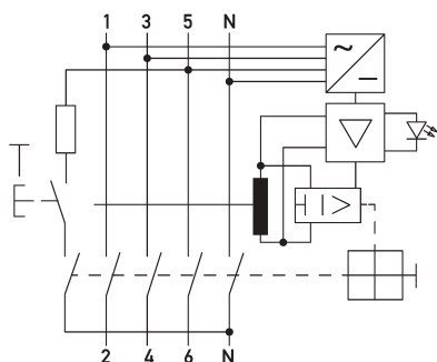
Schaltungsbeispiel Fehlerstromschutzschalter DFS 4 063-4/0,50-B SK R ISO HD
