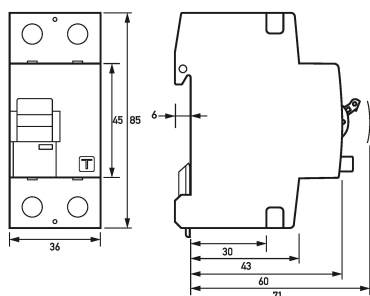
Maßzeichnung Fehlerstromschutzschalter DFS 2 063-2/0,50-A KV Hz60
