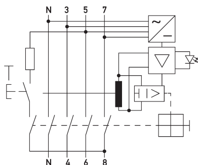
Schaltungsbeispiel Fehlerstromschutzschalter DFS 4 063-4/0,30-B SK S
