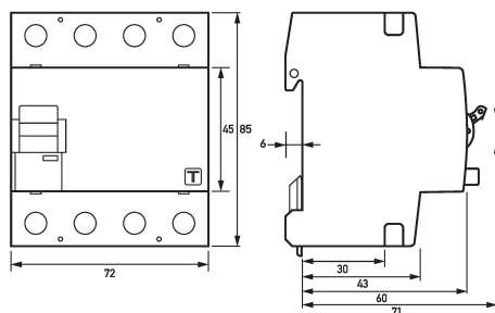
Maßzeichnung Fehlerstromschutzschalter DFS 4 063-4/0,30-B NK HD
