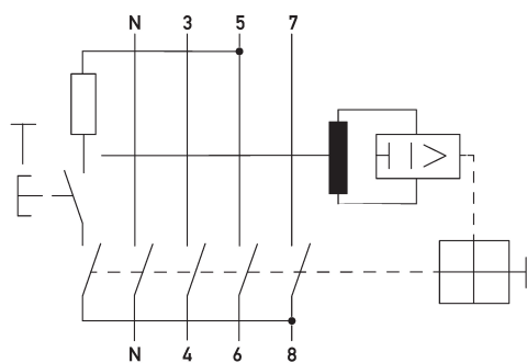
Schaltungsbeispiel Fehlerstromschutzschalter DFS 4 063-4/0,30-A S
