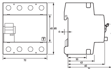
Maßzeichnung Fehlerstromschutzschalter DFS 4 063-4/0,30-A S
