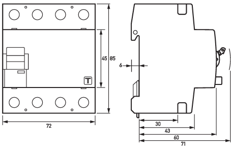
Maßzeichnung Fehlerstromschutzschalter DFS 4 063-4/0,30-B SK MI HD
