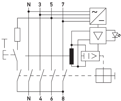
Schaltungsbeispiel Fehlerstromschutzschalter DFS 4 063-4/0,30-B SK MI HD
