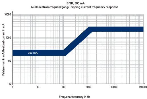
Diagramme Fehlerstromschutzschalter DFS 4 063-4/0,30-B SK MI HD
