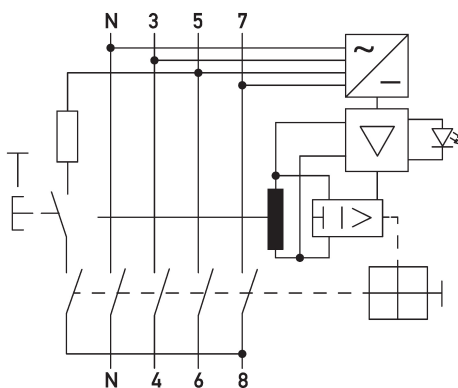
Esquema de conexiones DFS 4 B SK Hz V, 4 polos
