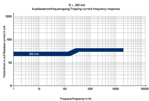
Diagramme Fehlerstromschutzschalter DFS 4 063-4/0,30-B+ MI
