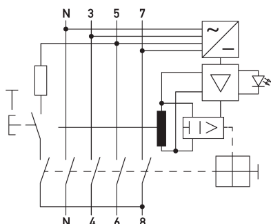
Schaltungsbeispiel Fehlerstromschutzschalter DFS 4 063-4/0,30-B NK Hz60 HD
