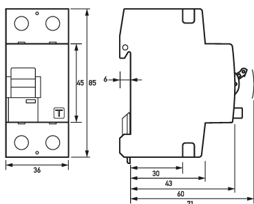
Maßzeichnung Fehlerstromschutzschalter DFS 2 063-2/0,30-A KV
