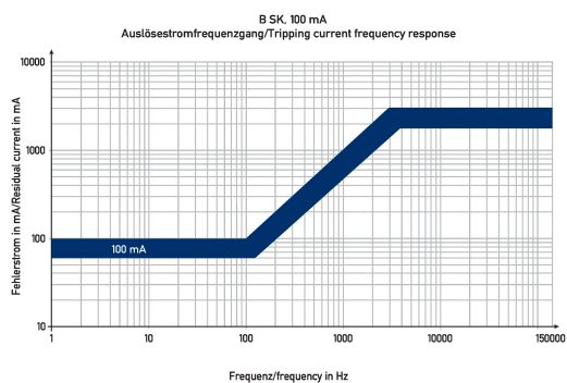
Diagramme Fehlerstromschutzschalter DFS 4 063-4/0,10-B SK
