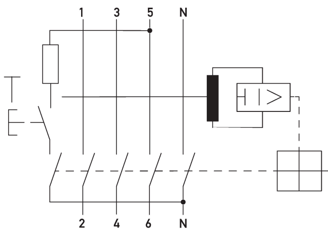
Anschlussschema DFS 4 A S, 4-polig N-rechts
