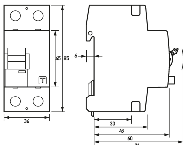
Maßzeichnung Fehlerstromschutzschalter DFS 2 063-2/0,10-B+
