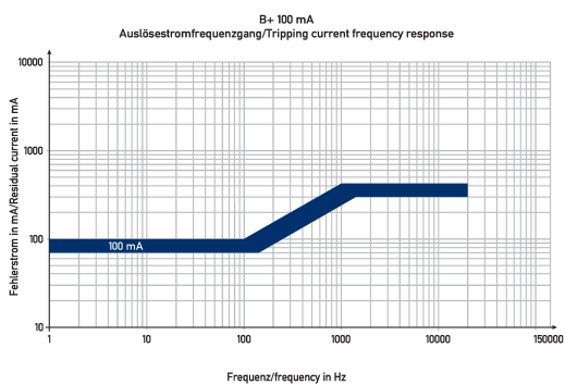
Diagramme Fehlerstromschutzschalter DFS 2 063-2/0,10-B+
