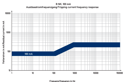
Diagramme Fehlerstromschutzschalter DFS 2 063-2/0,10-B NK
