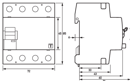
Maßzeichnung Fehlerstromschutzschalter DFS 4 063-4/0,03-A R V500
