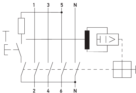
Schaltungsbeispiel Fehlerstromschutzschalter DFS 4 A VT, 4-polig
