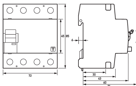
Maßzeichnung Fehlerstromschutzschalter DFS 4 A V T, 4-polig
