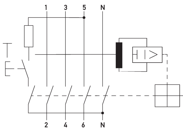
Esquema de conexiones DFS 4 A Hz, 4 polos N derecha
