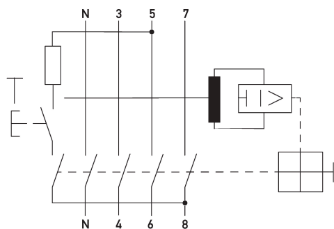
Schaltungsbeispiel Fehlerstromschutzschalter DFS 4 063-4/0,03-A KV Hz60 V500
