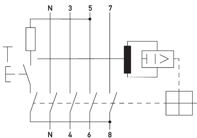
Esquema de conexiones DFS 4 A KV V, 4 polos
