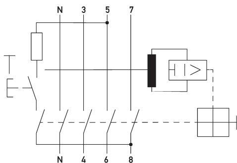
Schaltungsbeispiel Fehlerstromschutzschalter DFS 4 063-4/0,03-A KV V500
