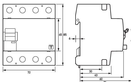
Maßzeichnung Fehlerstromschutzschalter DFS 4 063-4/0,03-A R HD
