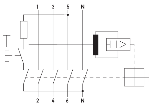
Schaltungsbeispiel Fehlerstromschutzschalter DFS 4 063-4/0,03-A R HD
