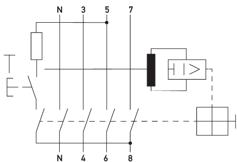
Schaltungsbeispiel Fehlerstromschutzschalter DFS 4 063-4/0,03-A
