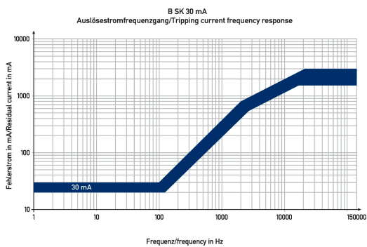
Diagramme Fehlerstromschutzschalter DFS 4 063-4/0,03-B SK Hz60 V127/220
