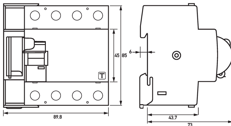
Maßzeichnung (Gruppenansicht)
