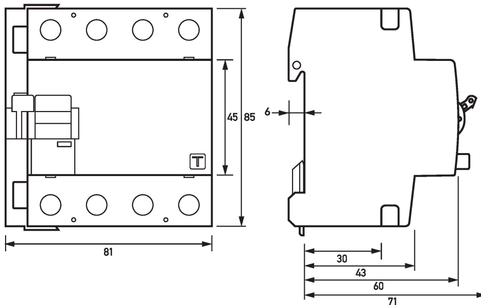
Maßzeichnung DFS 4 A EV NA HD, 4-polig (Gruppenansicht)
