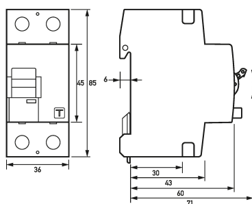
Dibujo acotado Interruptores diferenciales DFS 2 063-2/0,03-AC V110
