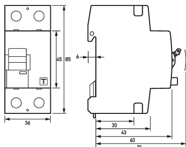
Maßzeichnung Fehlerstromschutzschalter DFS 2 063-2/0,03-A KV
