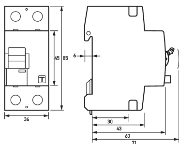
Dibujo acotado Interruptores diferenciales DFS 2 063-2/0,03-A
