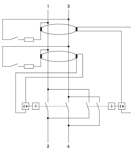
Ejemplo de cableado Interruptores diferenciales DFS 2 A KV Twin, 2 polos
