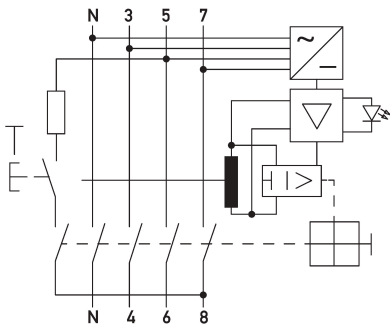
Ejemplo de cableado Interruptores diferenciales DFS 4 040-4/0,50-B SK
