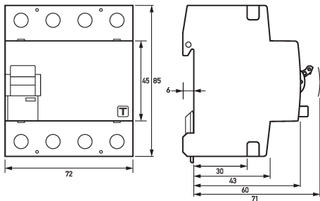
Dibujo acotado Interruptores diferenciales DFS 4 040-4/0,50-B SK
