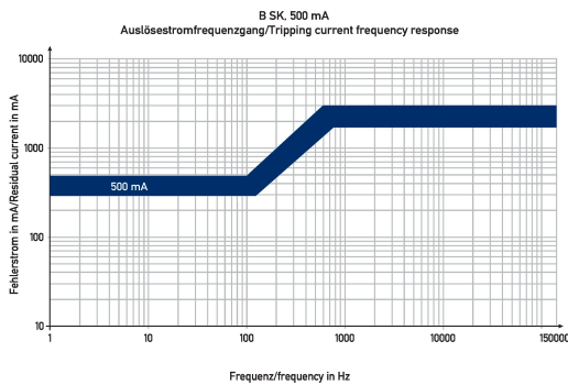
Diagramas Interruptores diferenciales DFS 4 040-4/0,50-B SK
