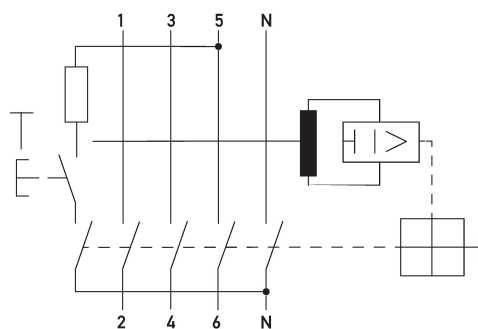
Ejemplo de cableado Interruptores diferenciales DFS 4 040-4/0,50-AC R Hz400
