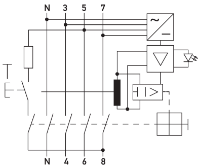
Anschlussschema
