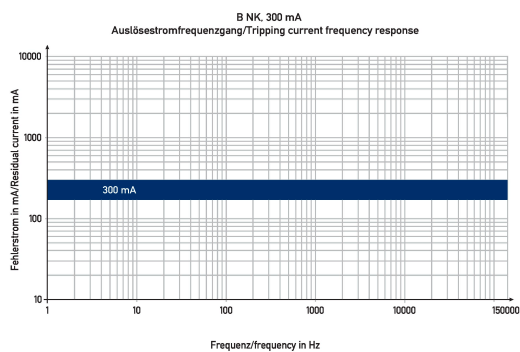
Diagramme Fehlerstromschutzschalter DFS 4 040-4/0,30-B NK HD
