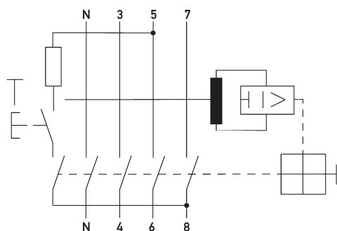
Ejemplo de cableado Interruptores diferenciales DFS 4 040-4/0,30-A HD
