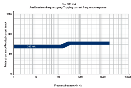
Curva característica B+ 300 mA
